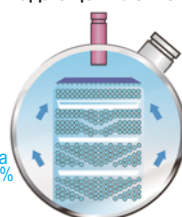
Испаритель со сплошной падающей пленкой
