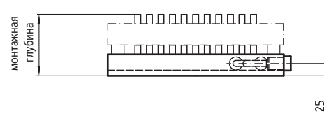
Подключение боковое слева (под.труб. внутри), вентиль вверху справа
