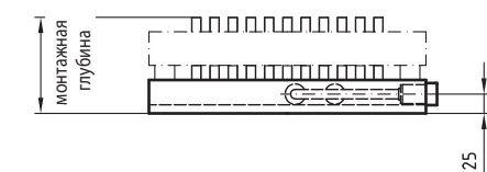
Подключение боковое справа (под.труб. внутри), вентиль внизу справа
