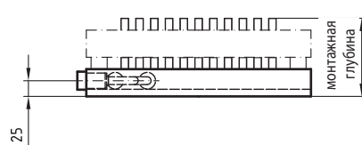
Подключение боковое слева (под.труб. внутри), вентиль вверху слева
