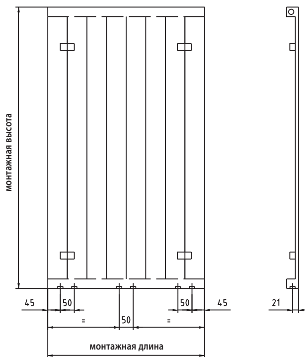
схема подключений 69/89/98
