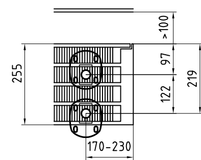
Монтаж перед стеклом Тип: KSN55 + KSV55
