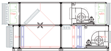
Приточно-вытяжная установка с пластинчатым рекуператором и смесительной секцией (вертикальное исполнение)
