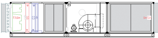
Приточная установка, шумоглушители 1050, 1450, 1950 мм для входящего и выходящего воздуха
