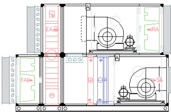
Приточно-вытяжная установка с роторным рекуператором (вертикальное исполнение) и секцией смешения
