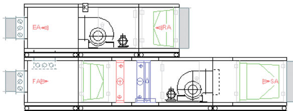
Приточно-вытяжная установка со смешивательной секцией (вертикальное исполнение), длинный карманный фильтр F5-F9
