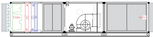
Приточная установка, шумоглушители 750, 1050, 1450, 1950 мм для входящего и выходящего воздуха
