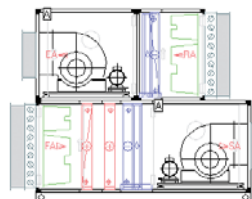
Приточно-вытяжная установка с гликолевым теплоутилизатором
