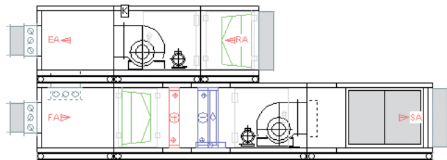
Приточно-вытяжная установка со смешивательной секцией (вертикальное исполнение), шумоглушитель 880 или 1380 мм на входе и выходе
