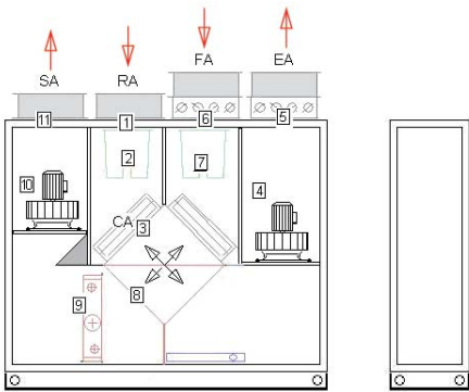
Приточно-вытяжная конфигурация с нагреванием, тип x10
