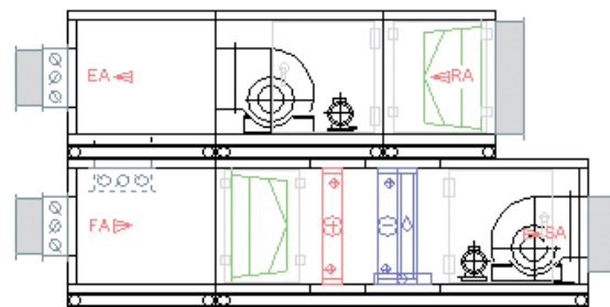
Приточно-вытяжная установка со смешивательной секцией (вертикальное исполнение)
