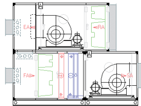
Приточно-вытяжная установка с секцией смешения (вертикальное исполнение)
