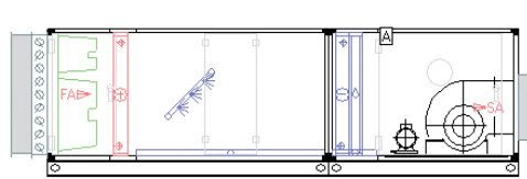
Приточная установка с камерой парового увлажнения
