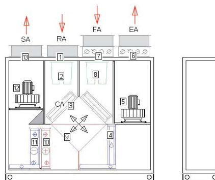
Приточно-вытяжная конфигурация, нагревание и охлаждение и выпрямление, тип x12-E, x13-E
