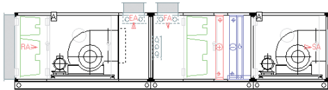
Приточно-вытяжная установка с секцией смешения в линию
