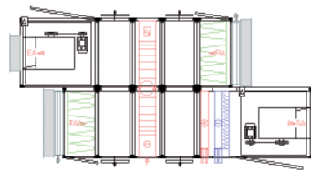
Приточно-вытяжная установка с роторным рекуператором (горизонтальное исполнение)
