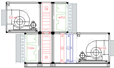
Приточно-вытяжная установка с роторным рекуператором (вертикальное исполнение)
