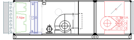
Приточная установка, газонагреватель
