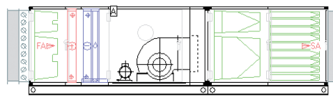
Приточная установка, длинный карманный фильтр F5-F9, угольный фильтр
