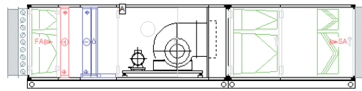
Приточный агрегат, длинный карманный фильтр F7, угольный фильтр, фильтр HEPA H10-H13
