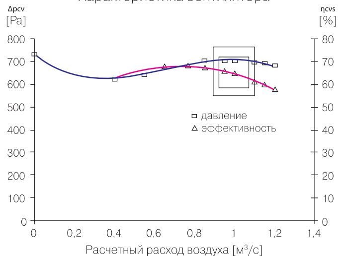
Характеристика вентилятора
