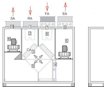
Приточно-вытяжная конфигурация с выпрямителем, тип x00-E
