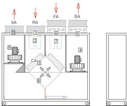
Приточно-вытяжная конфигурация, тип x00
