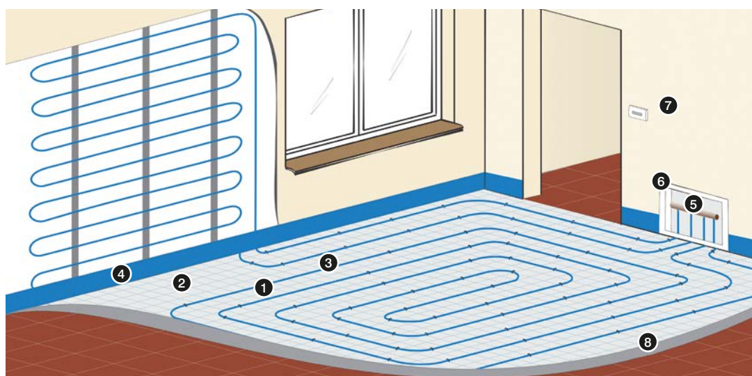
Рис. 46. Элементы панельно-лучистого отопления/охлаждения KAN-therm
