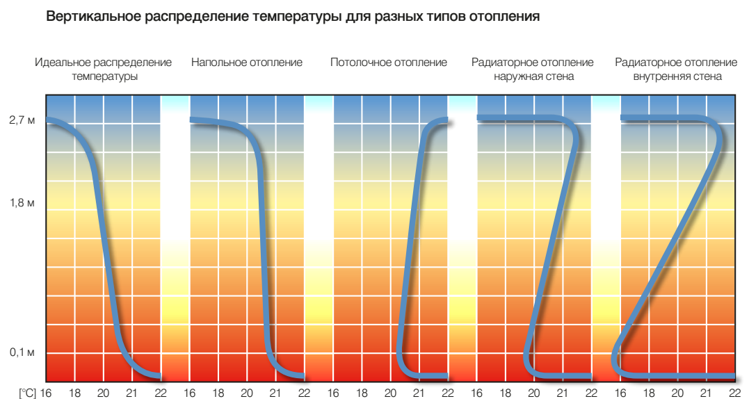
Рис. 1. Вертикальное распределение температуры для разных типов отопления
