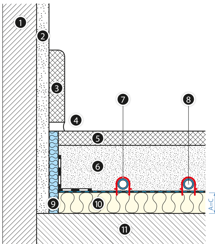
Рис. 21. Напольный отопительный прибор с пенополистирольной плитой KAN-therm Tacker на перекрытии над внутренним помещением
