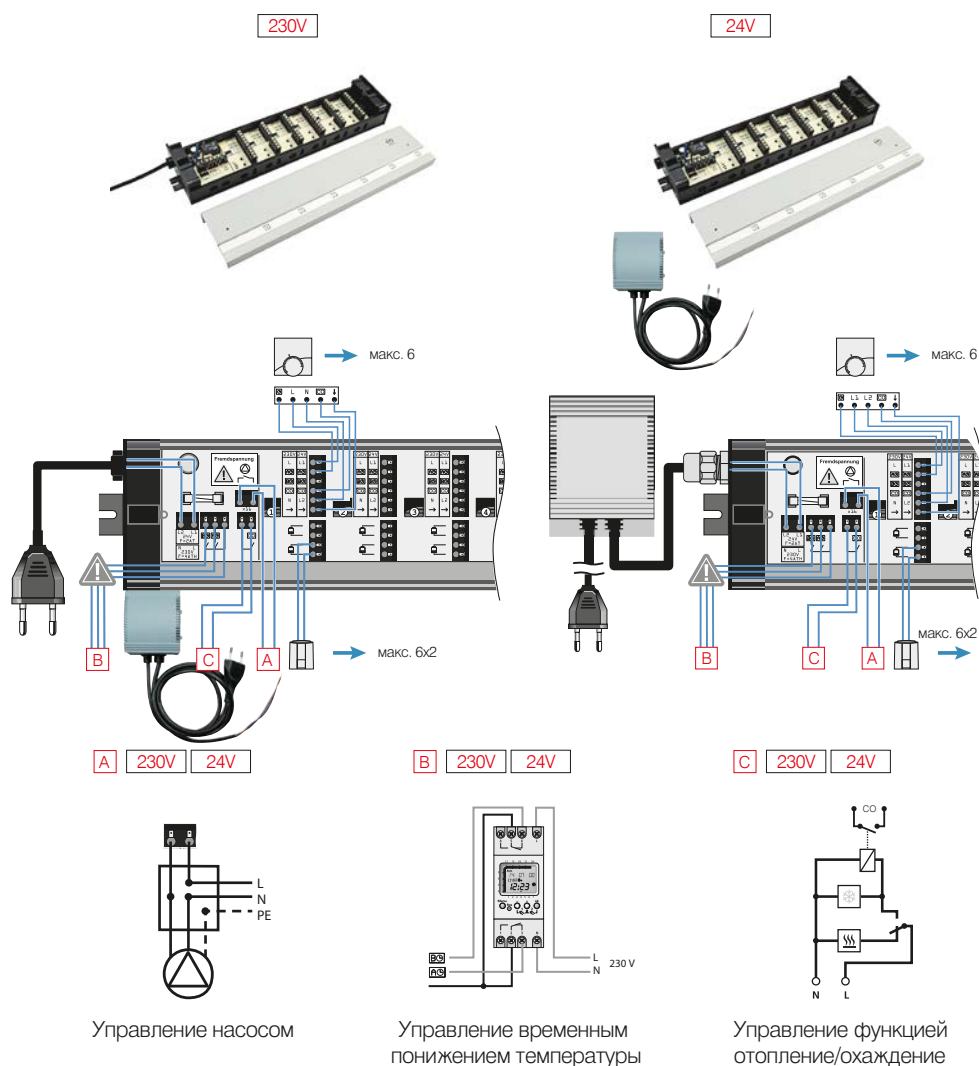
Рис. 71. Конфигурация клеммной колодки Basic 230 В или 24 В отопление/охлаждение с насосным модулем
