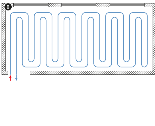
Рис. 8. Контур напольного отопления/охлаждения двойной меандр.
