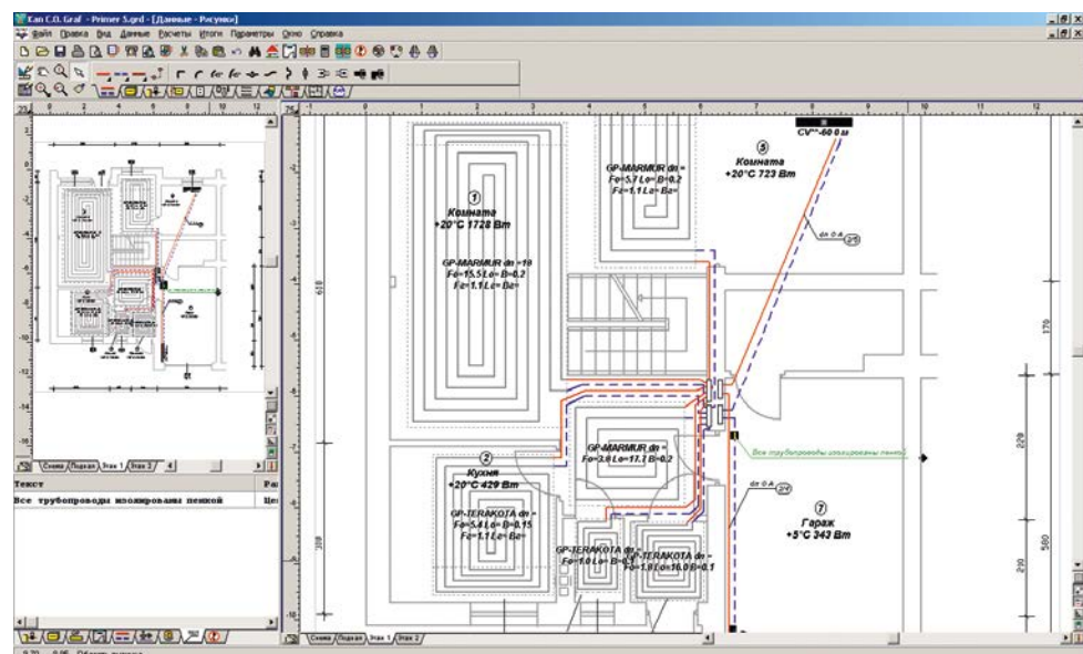
Рис. 81. План этажа с нанесенными напольными отопительными приборами.
