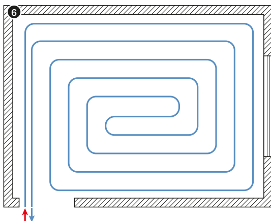
Рис. 6. Контур напольного отопления/охлаждения в форме спирали (улитки).
