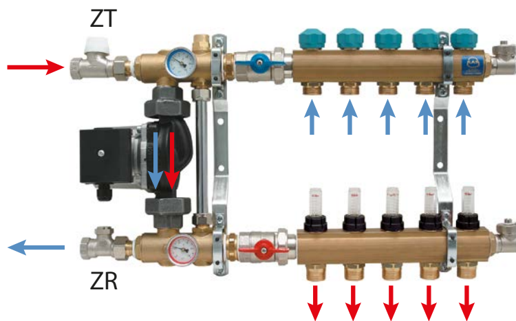
Рис. 60. Коллекторная группа со смесительной системой серии 77A (или 73A) – направления потоков воды
