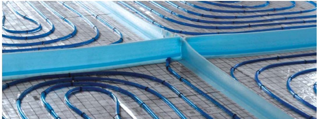
Рис. 13. Деление греющей поверхности разделительными швами
