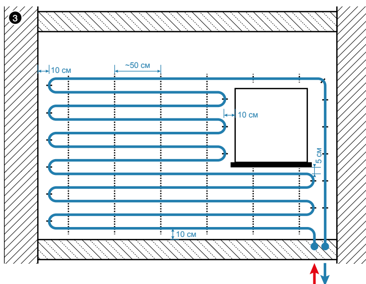
3. Монтажные расстояния в стеновом отоплении
