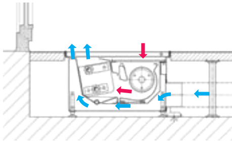
Разрез (пример с роллонной решеткой)
