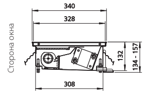
Разрез (пример с рулонной решеткой)
