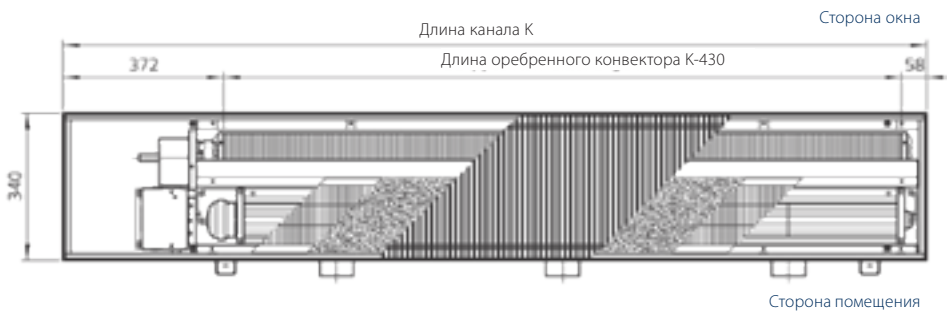
Вид сверху (Katherm НК 340 с функцией подачи приточного воздуха, высота канала 190 мм)
