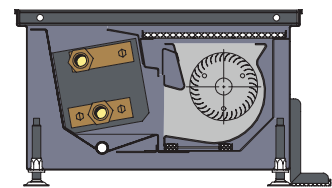
Katherm HK 340, высота канала 190 мм, 2-трубная система
