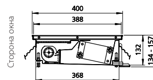
Разрез (пример с рулонной решеткой)
