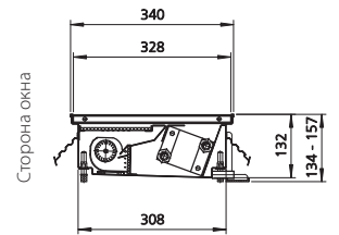
Разрез (пример с рулонной решеткой)
