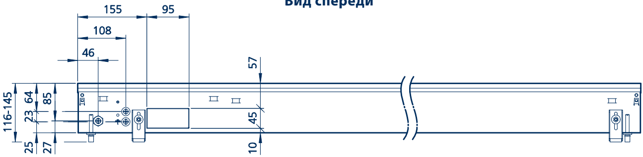
Вид спереди
