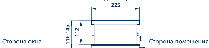
Вид сбоку
