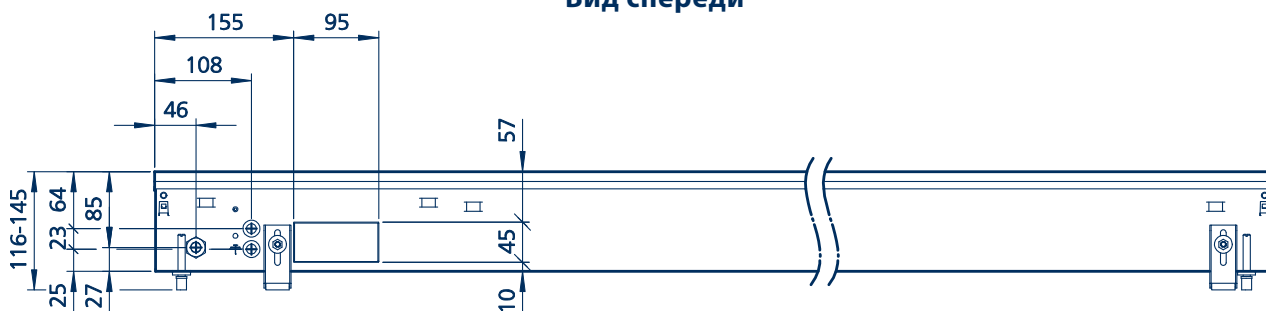
Вид спереди
