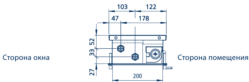
Вид А-А
