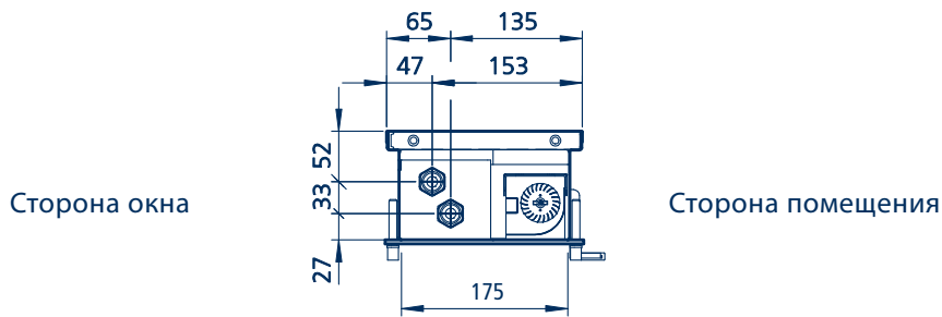
Вид А-А
