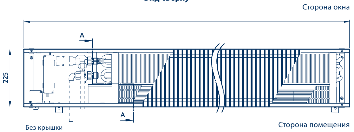
Вид сверху
