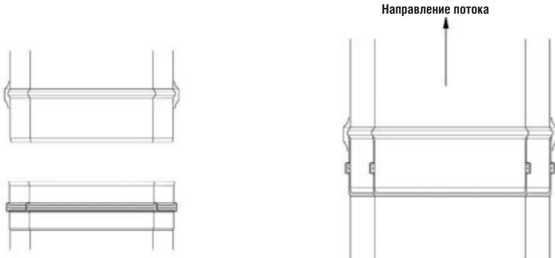
Рис. 3 Трубное соединение
