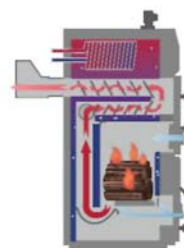
Дровяная топка Biotriplex
