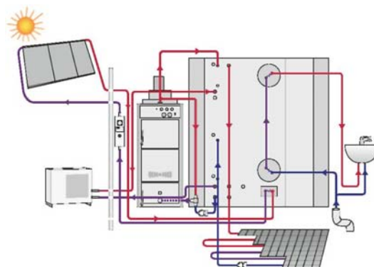
На примере, подключение контура солнечной энергии и теплового насоса воздух-вода к системе твердотопливного отопления.
