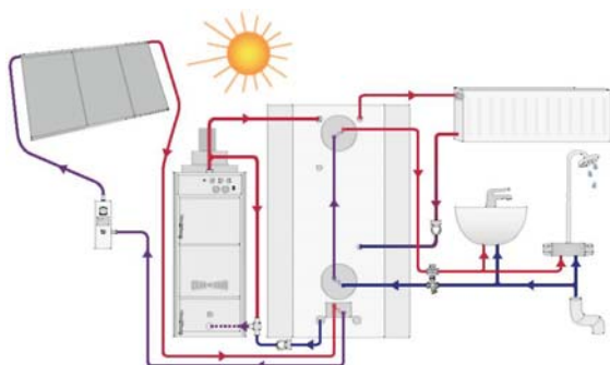
Твердотопливный котел Econature всегда подключается к аккумулятору энергии. На примере, аккумулятор Ovali, подключенный к контуру солнечной энергии.
