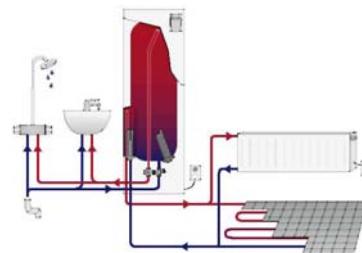
В Tehowatti объединены электрокотел и водонагреватель.
