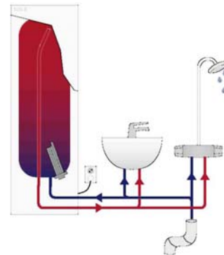
VLM нагревает ГВС.
