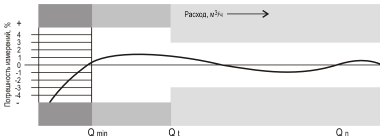
Типичная кривая погрешностей измерений (соответствует теплосчетчикам «Sensonic» компактный и комбинационный 0,6; 1,5; 2,5)
