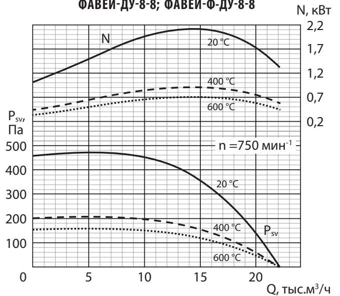
ФАВЕЙ-ДУ-8-8; ФАВЕЙ-Ф-ДУ-8-8
