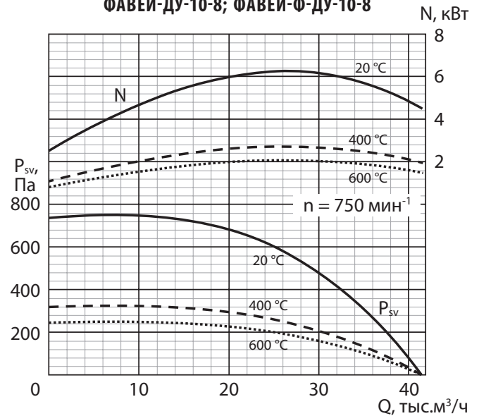
ФАВЕЙ-ДУ-10-8; ФАВЕЙ-Ф-ДУ-10-8
