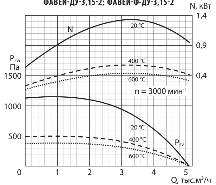
ФАВЕЙ-ДУ-3,15-2; ФАВЕЙ-Ф-ДУ-3,15-2
