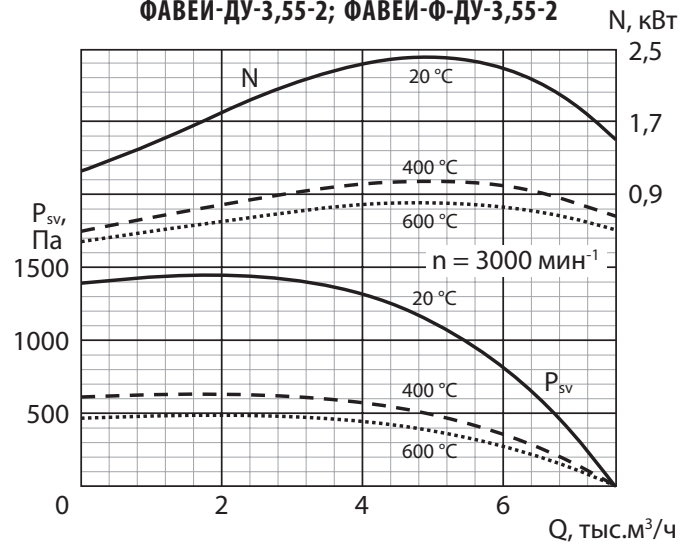
ФАВЕЙ-ДУ-3,55-2; ФАВЕЙ-Ф-ДУ-3,55-2
