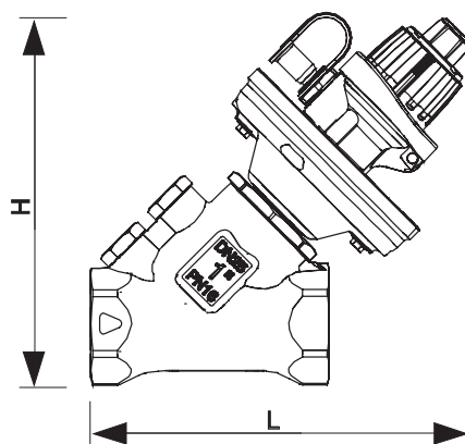
Рис. 2 Вид сбоку
