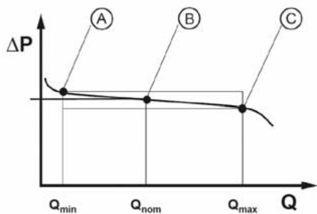
Рис. 6 Регулировочная характеристика
