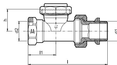
Рис. 2. Прямой с внутренним резьбовым соединением на входе.
