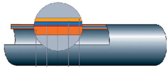
Наружный слой - полиэтилен PE-X или PE-HD белого цвета. Слой клея. Алюминиевая труба – с продольным сварным швом. Слой клея. Внутренний слой - полиэтилен PE-Xc или PE-RT белого цвета.
