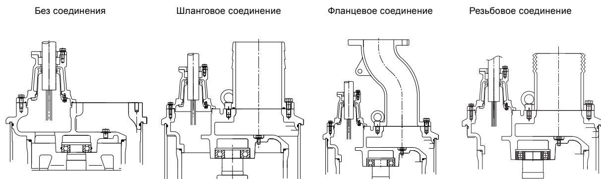
Рис. 4 Напорные соединения
