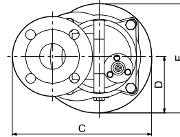
Фланцевое соединение
