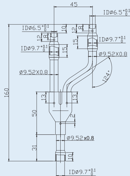
Жидкостная труба
