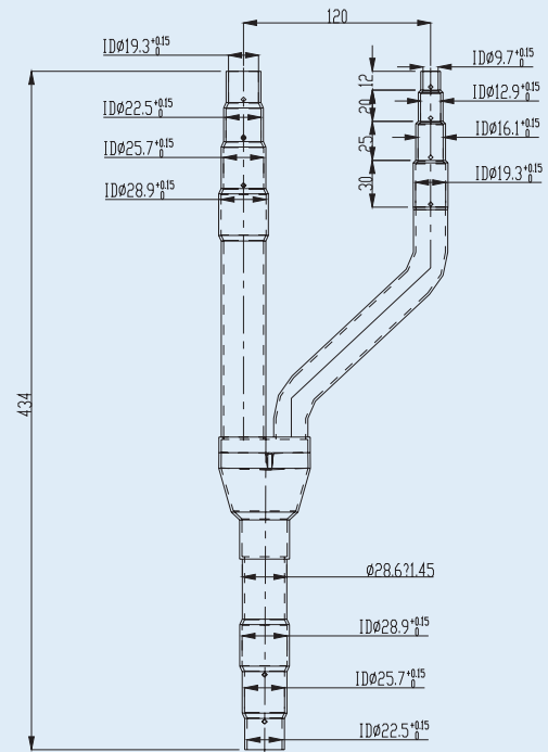
Жидкостная труба
