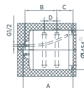
(1) TGU 200 N: диаметр 500 мм, глубина 507 мм
