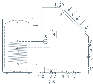
КGV 300-1 с коллектором солнечной энергии
