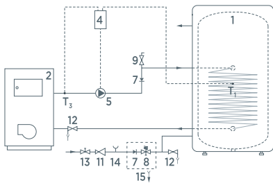
КGV 200-1 с котлом центрального отопления
