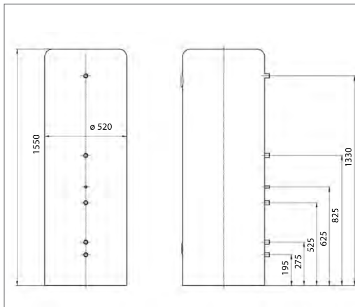
Габаритные размеры
