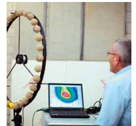
Источник шума может быть точно определен с помощью акустической камеры.
