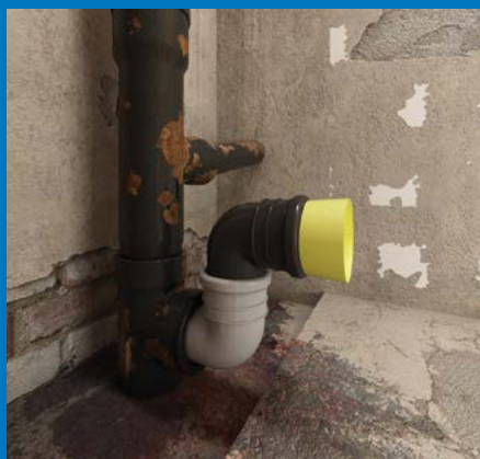
Монтажный элемент может быть присоединен к любому типу канализационного отвода.
