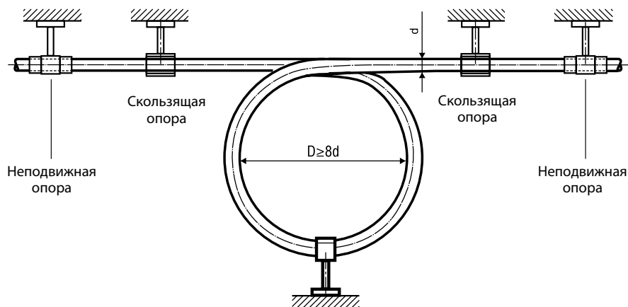
Рисунок 4. Петлеобразный компенсатор
