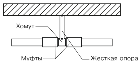
Рисунок 13. Неподвижная опора, выполненная хомутом между муфт
