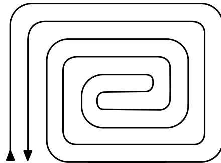
Рисунок 26. Укладка теплого пола спиралью
