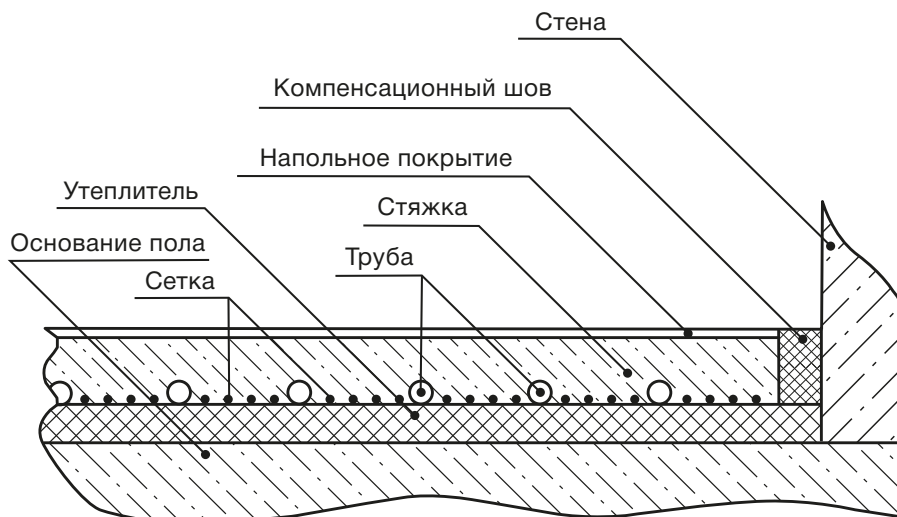
Рисунок 24. Схема устройства системы «Теплый пол»
