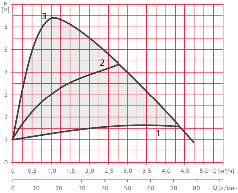
Пропорциональное давление
