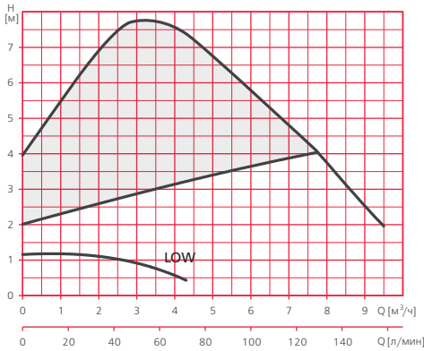
Пропорциональное давление
