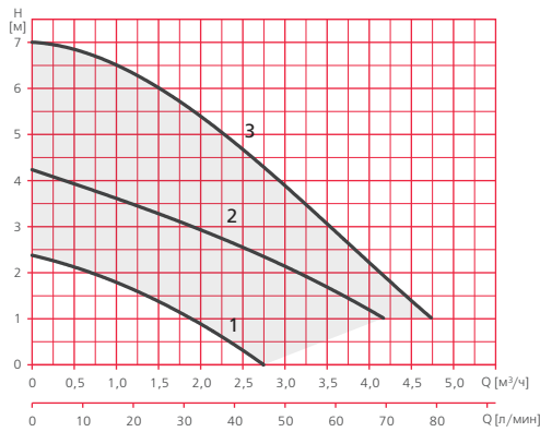
Постоянная скорость
