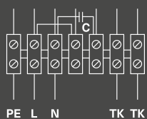
Схема 2 (230 В, 1 ф, 50 Гц.)
