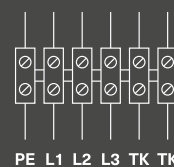
Схема 3 (400 В, 3 ф, 50 Гц.)
