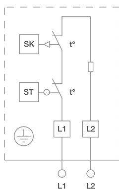
Схема 2 (400 В, 2 фазы)
