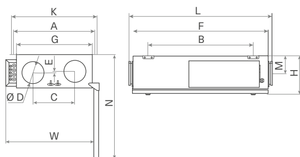
CPE 1500
