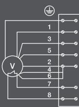
Схема 4 (400 В, 3 ф.)
