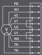
Схема 3 (Δ — 400 В, 3 ф.)
