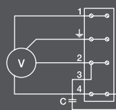
Схема 5 (230 В, 1 ф.)
