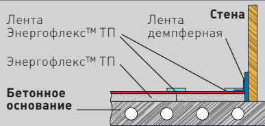
Схема установки тёплого пола
