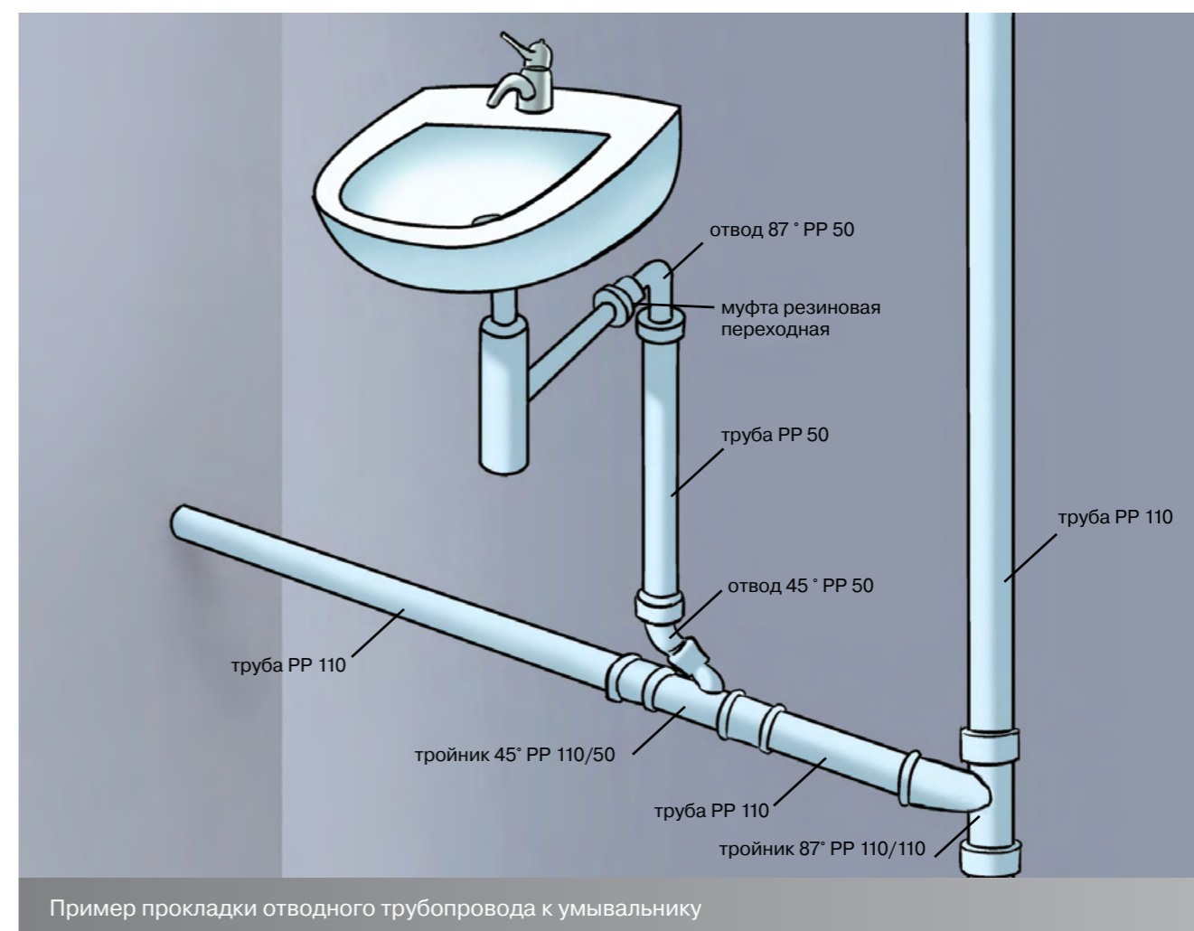
Принципиальная схема внутренней канализации
