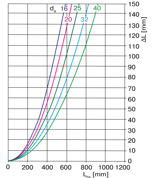
Определение длины плеча компенсатора
