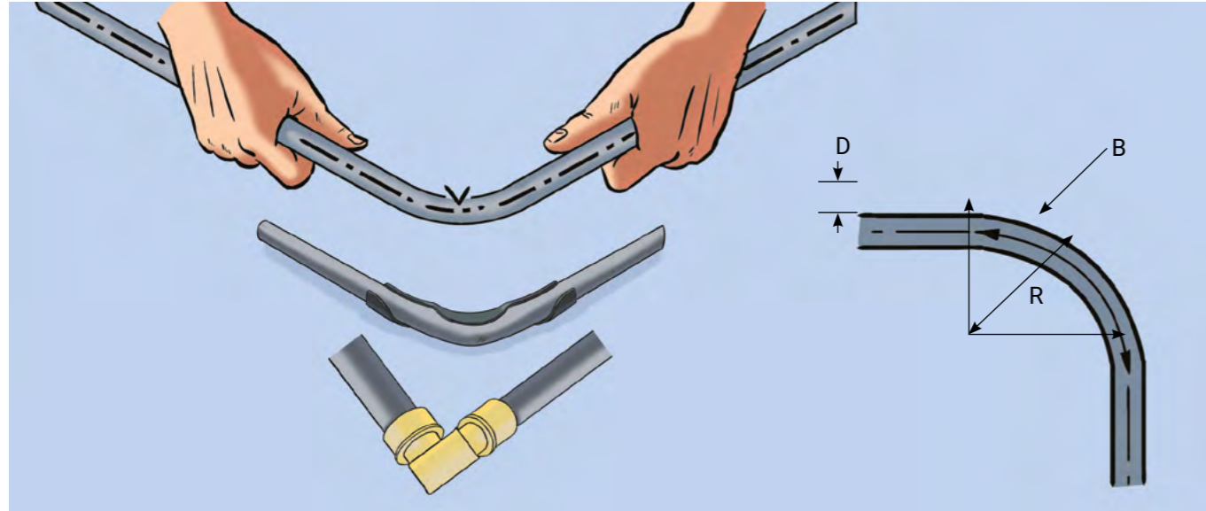
Минимальный радиус изгиба при изгибании вручную ( R = 8 \times D )
