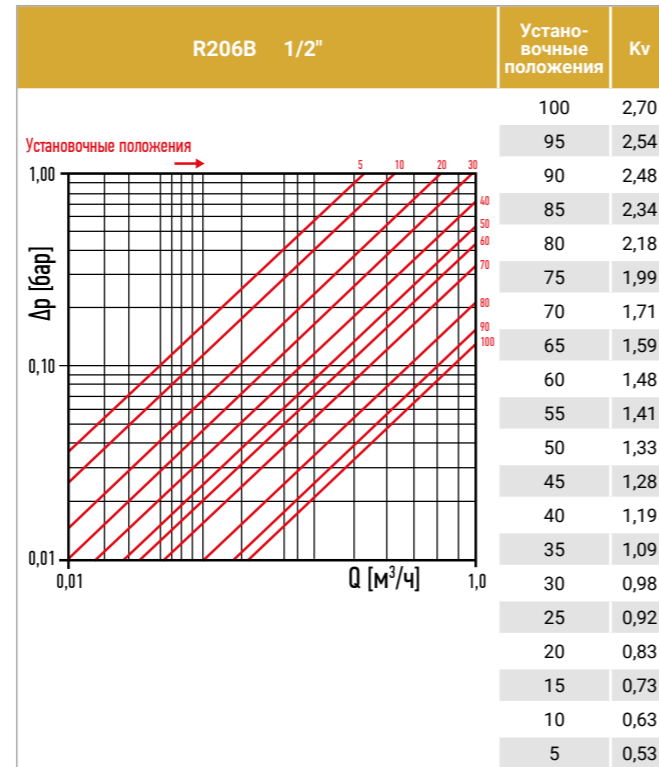
Диаграмма зависимости потерь давления от расхода для клапана партнера
