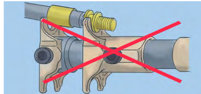
При запрессовке фитинг с гильзой перекошены (несоосность) либо зажаты между губок под углом
