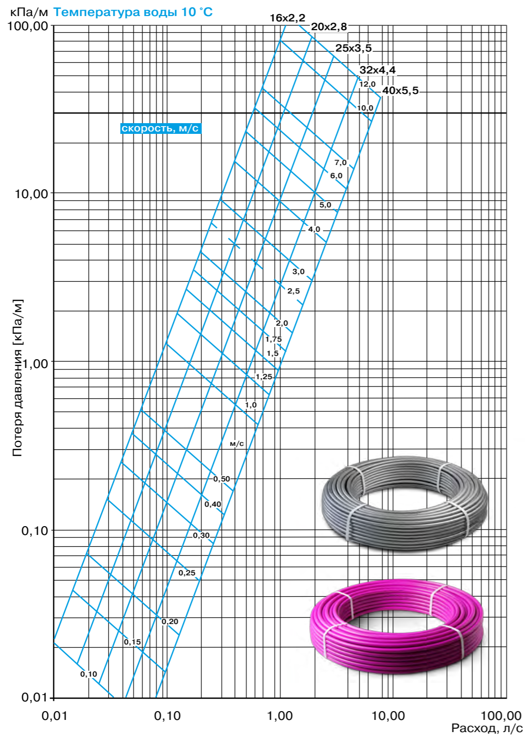
График линейных потерь давления в трубах PRO AQUA PE-Ха (серебристая) SDR 7.4 и PE-RT SDR 7.4 (фиолетовая)
