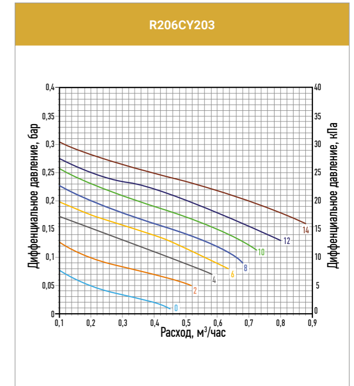
Для установки требуемого перепада давления необходимо воспользоваться диаграммами и таблицами настроек.
