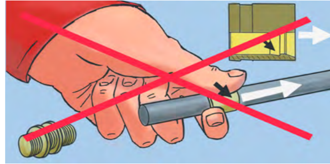
Гильза надета «не той стороной»: фаска внутри гильзы направлена в противоположную сторону от фитинга
