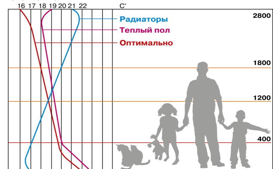
График распределения тепла (для помещения с высотой потолка 2.8 м)
