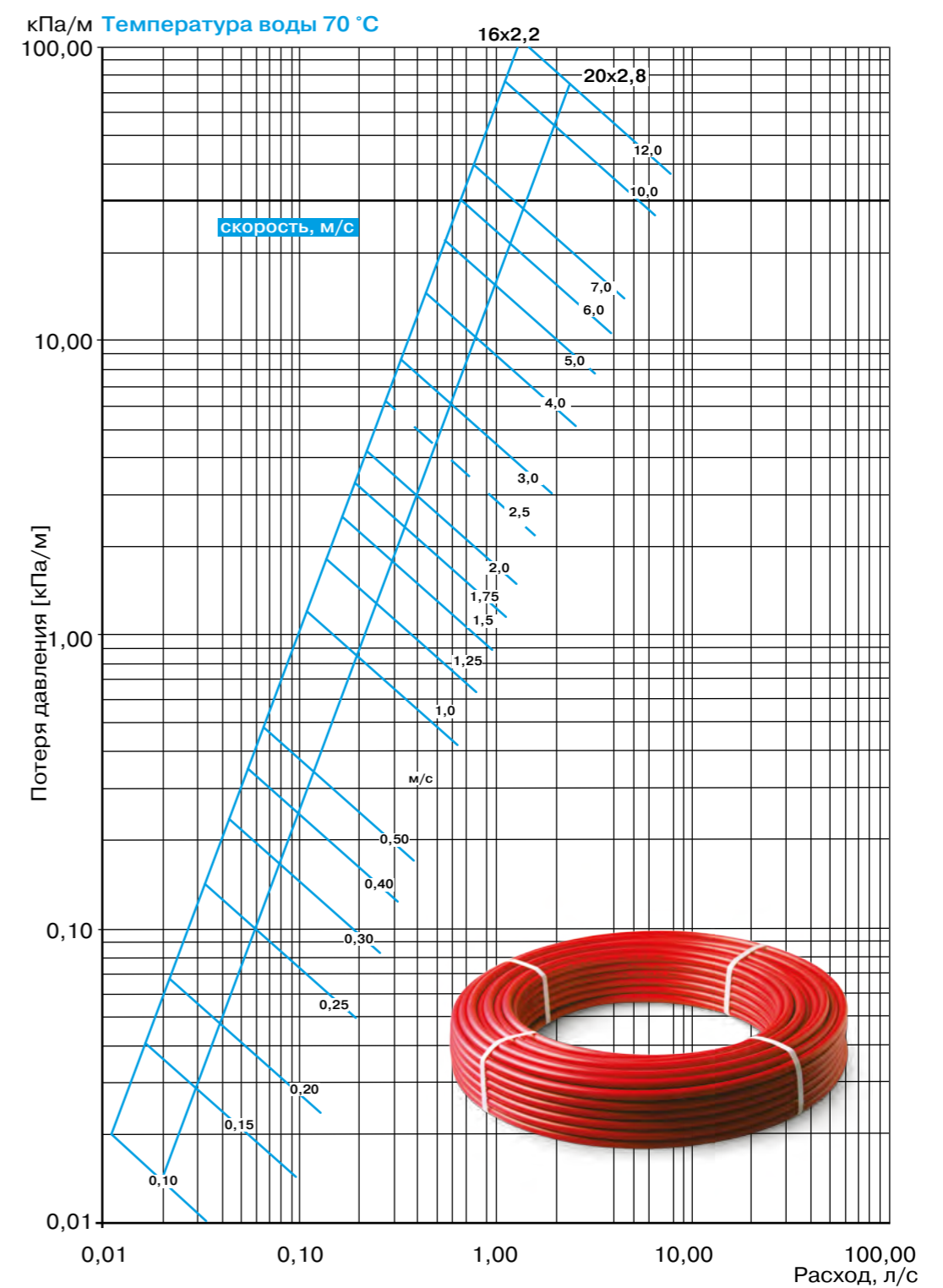
График линейных потерь давления в трубах PRO AQUA PE-Ха (красная), S3.5 / S4.5
