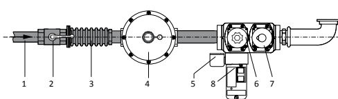
VCS Kromschröder
