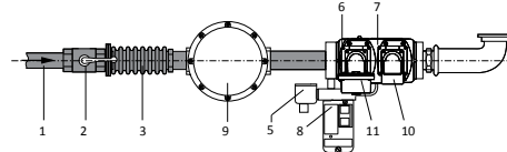
VGD Siemens
