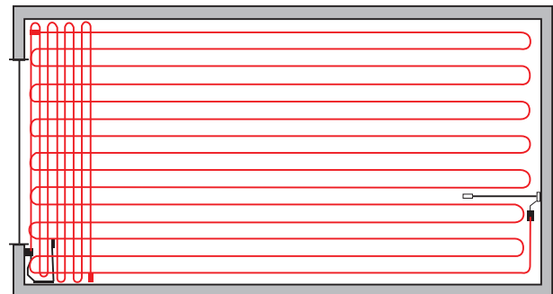
Пример раскладки нагревательных кабелей с дополнительным обогревом в краевой зоне.
