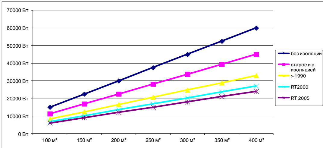
График для наружной T^{\circ} = -10^{\circ}\text{C} и комнатной температуры 20^{\circ}\text{C} (для Франции)
