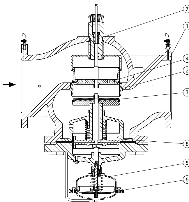
Устройство клапана АВ-QM Д y = 200, 250 мм
