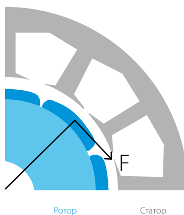
Обычный двигатель с внутренним ротором
