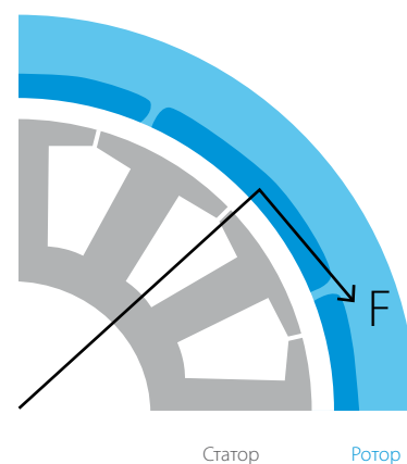
Внешний ротор Daikin
