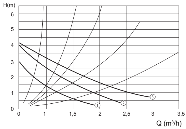
GHN 25/70-130
