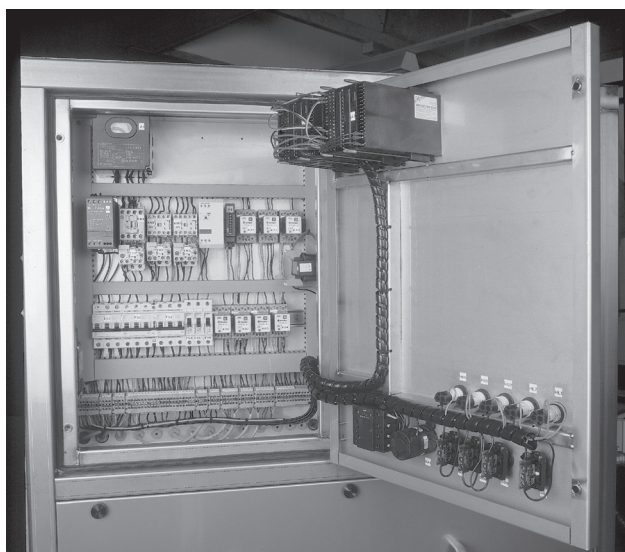
Газораспределительная секция осушителя типа G
