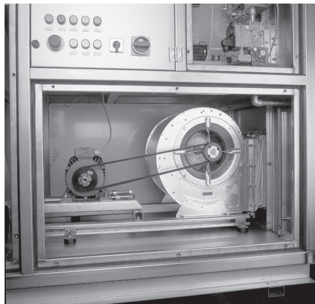
Секция ротора
