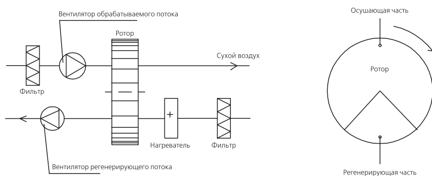
Рис. 2. Принципиальная схема осушителей CR100 ... CR300
