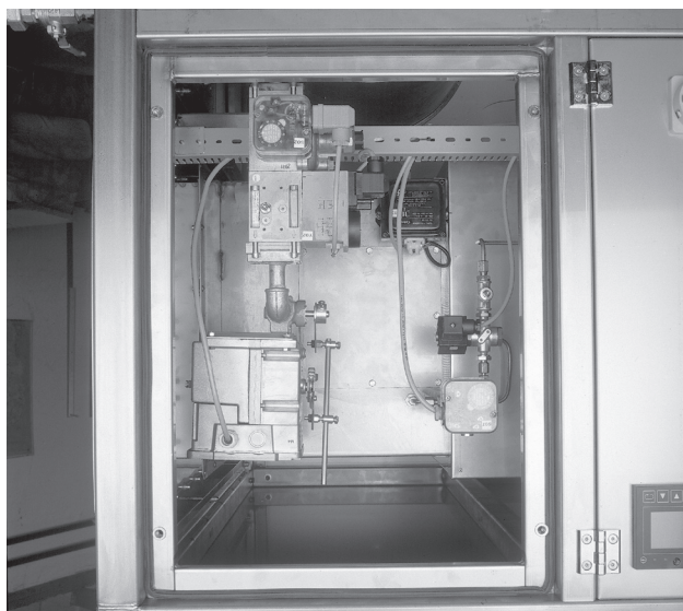
Секция вентилятора
