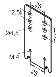
Удлинительная скоба
