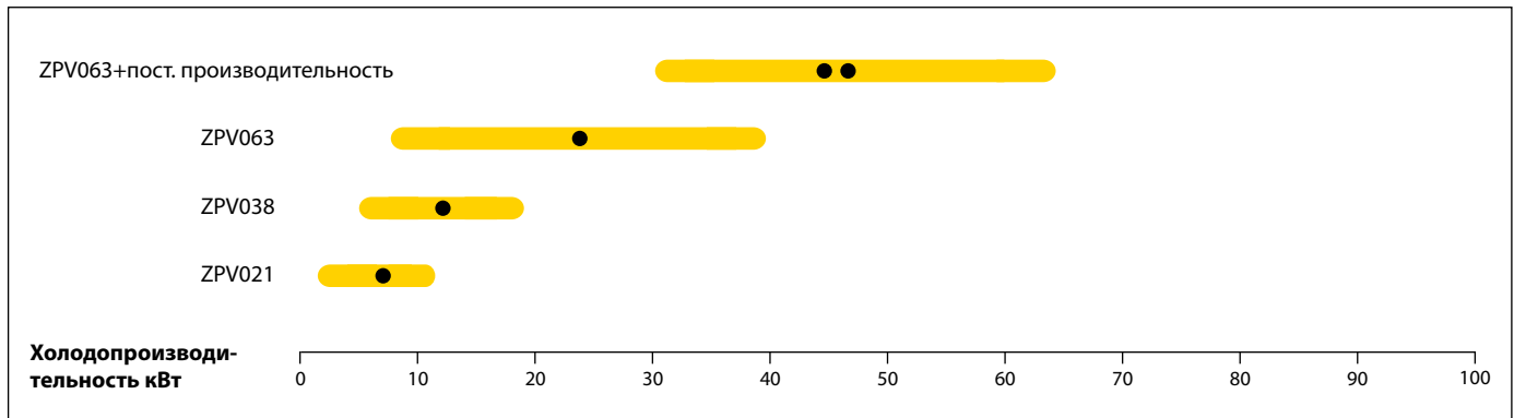
Copeland Scroll™ ZPV063 Компрессор с регулируемой скоростью и приводом
