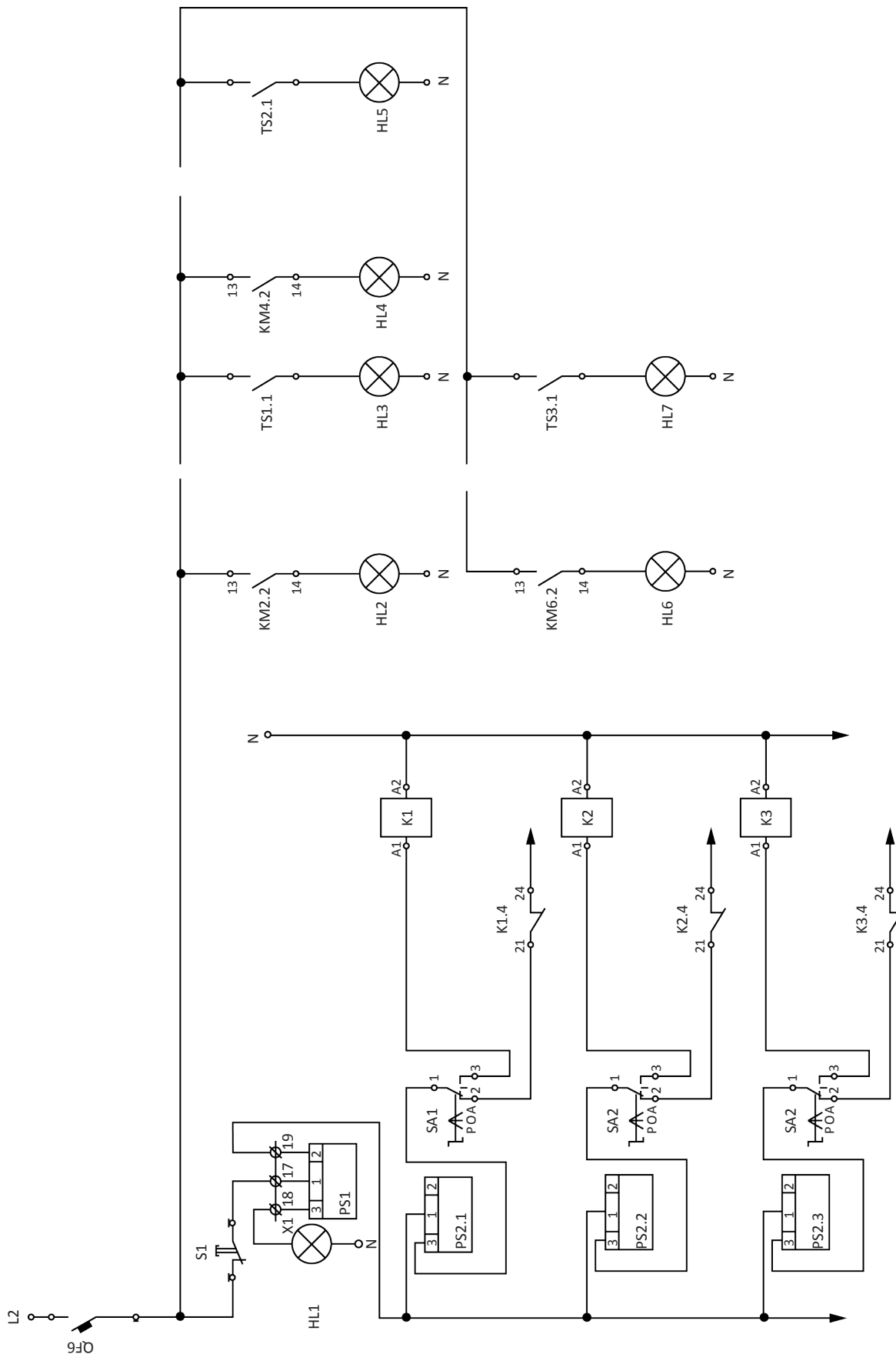
Схема RCC – релейно-каскадное регулирование (3 насоса)
