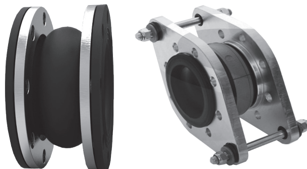
Рис. 11 Компенсаторы с ограничительными стяжками и без них
