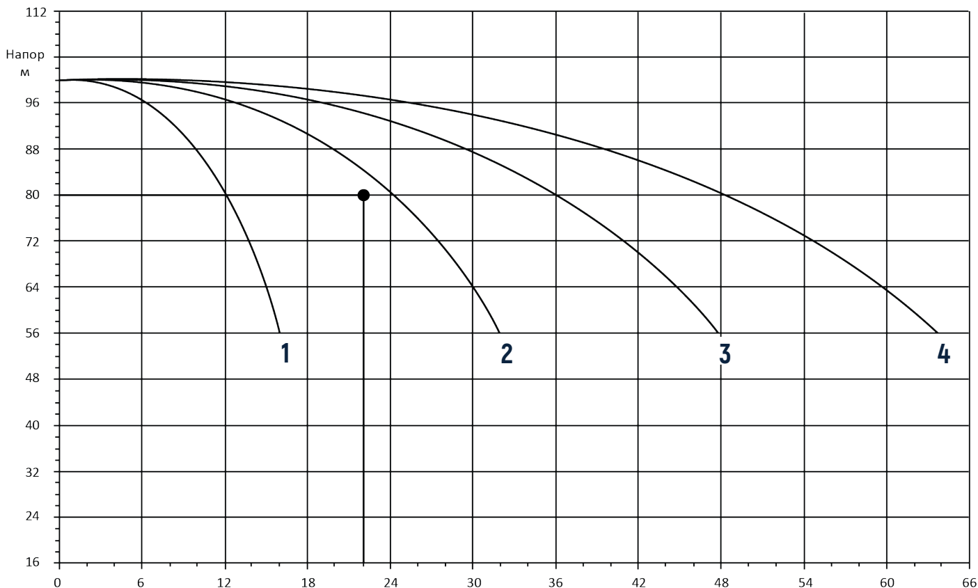
Рис. 13 Пример выбора насосной установки CNP PBS 2 CDL 12-8 50 Гц, ISO 9906 класс 3
