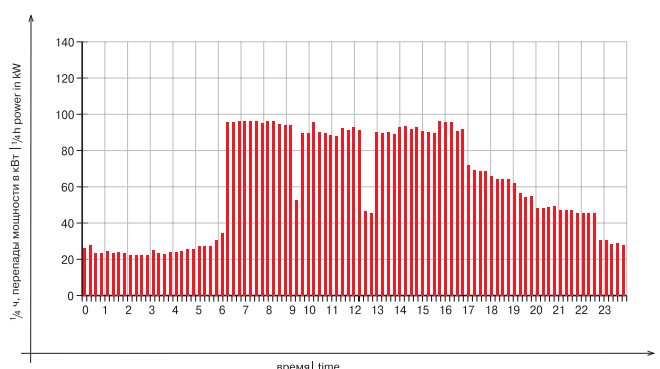
Колебания мощности при использовании регулятора LA-4G 46592 | Solution with LA-4G 465 92: Power peaks limited to 100 kW
