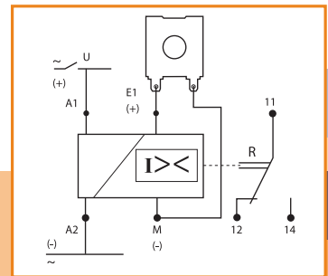
Схема подключения MRIH 400
