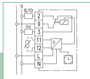
Схема подклю÷ения | Wiring diagram
