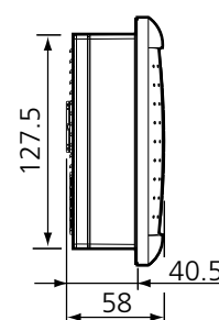
Монтаж в панель
