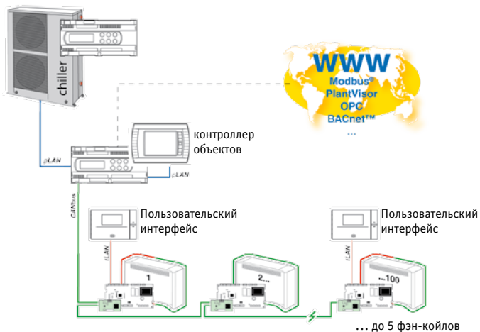
multimaster e-drobus
