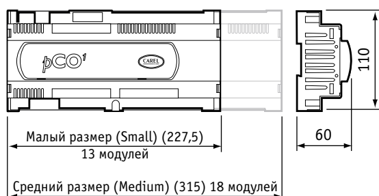
Габаритные размеры, мм
