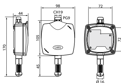
Габаритные размеры, мм
