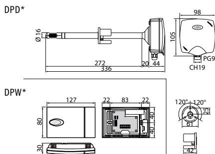
Габаритные размеры, мм
