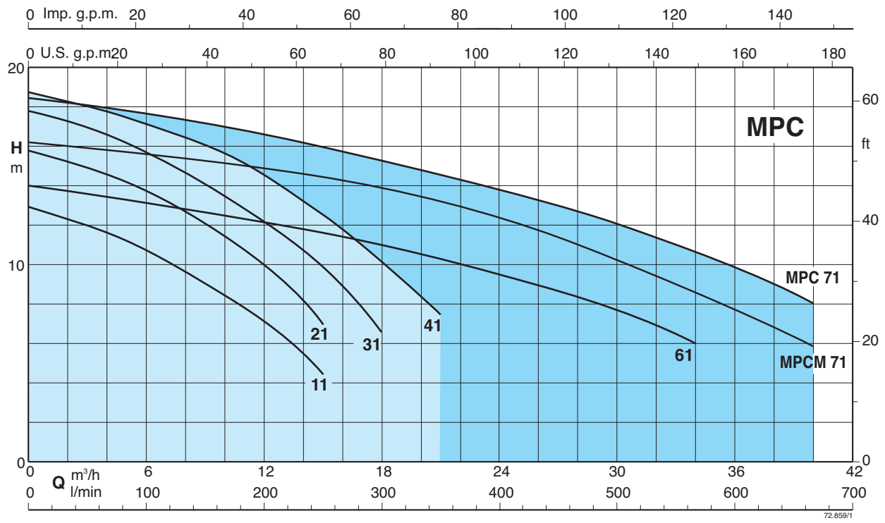
Coverage chart - Campo de aplicaciones n ≈ 3450 rpm
