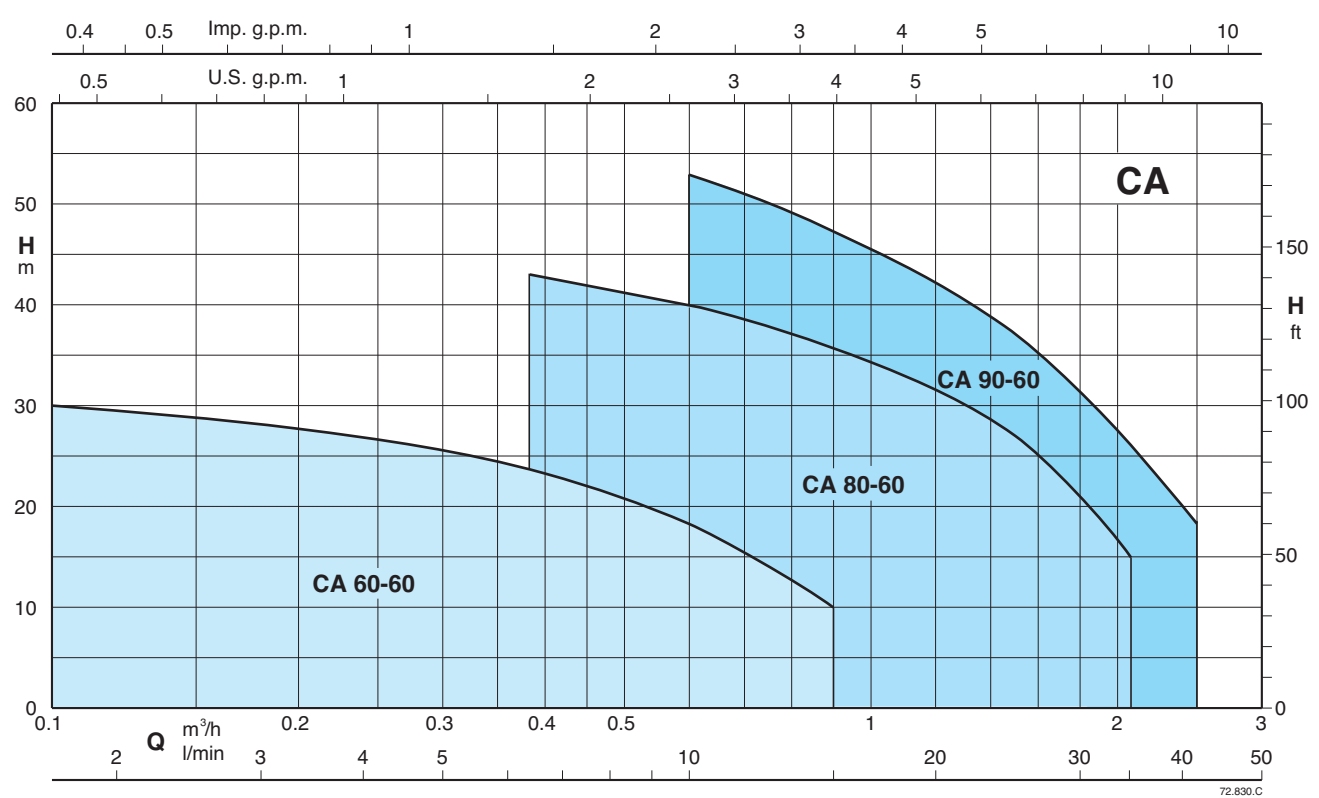
Coverage chart - Campo de aplicaciones n ≈ 3450 rpm
