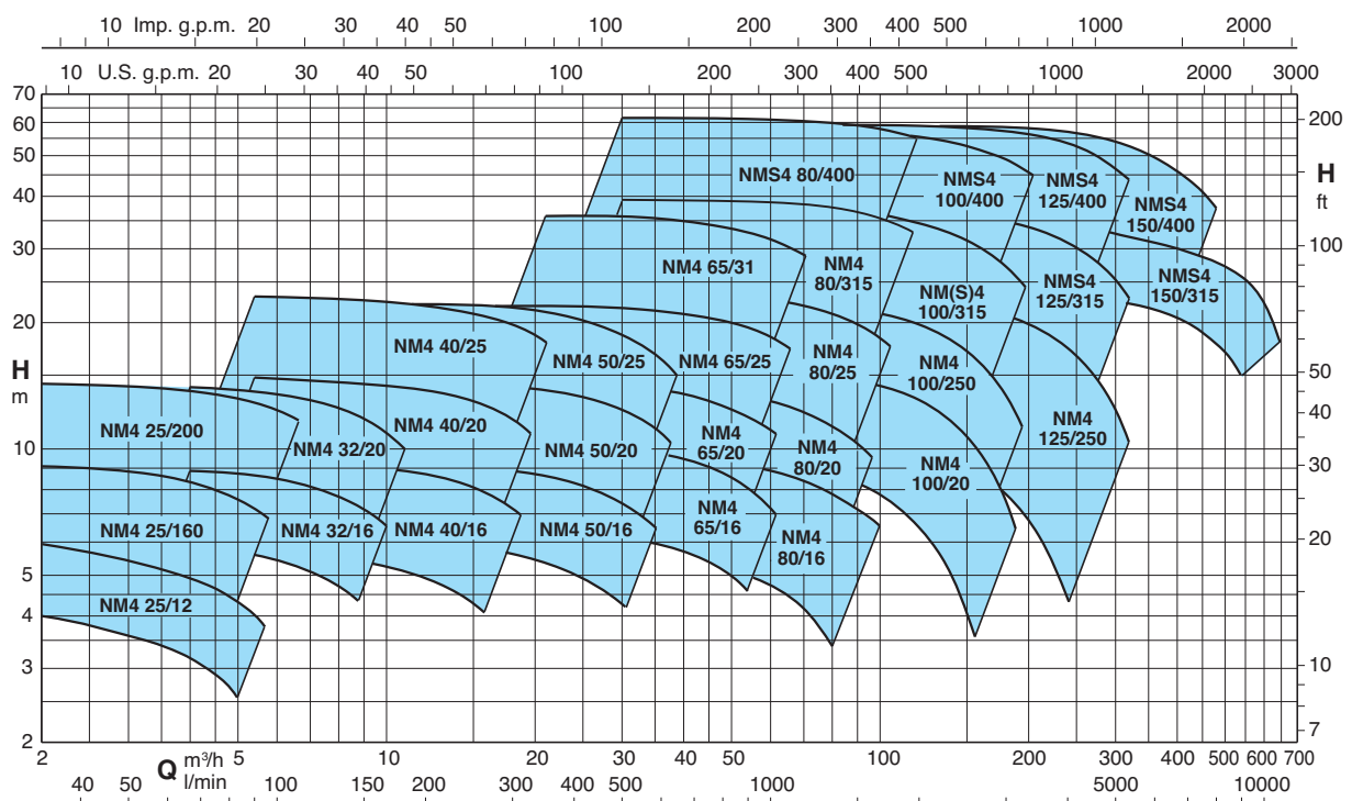
Coverage chart - Campo de aplicaciones n \approx 1750 rpm
