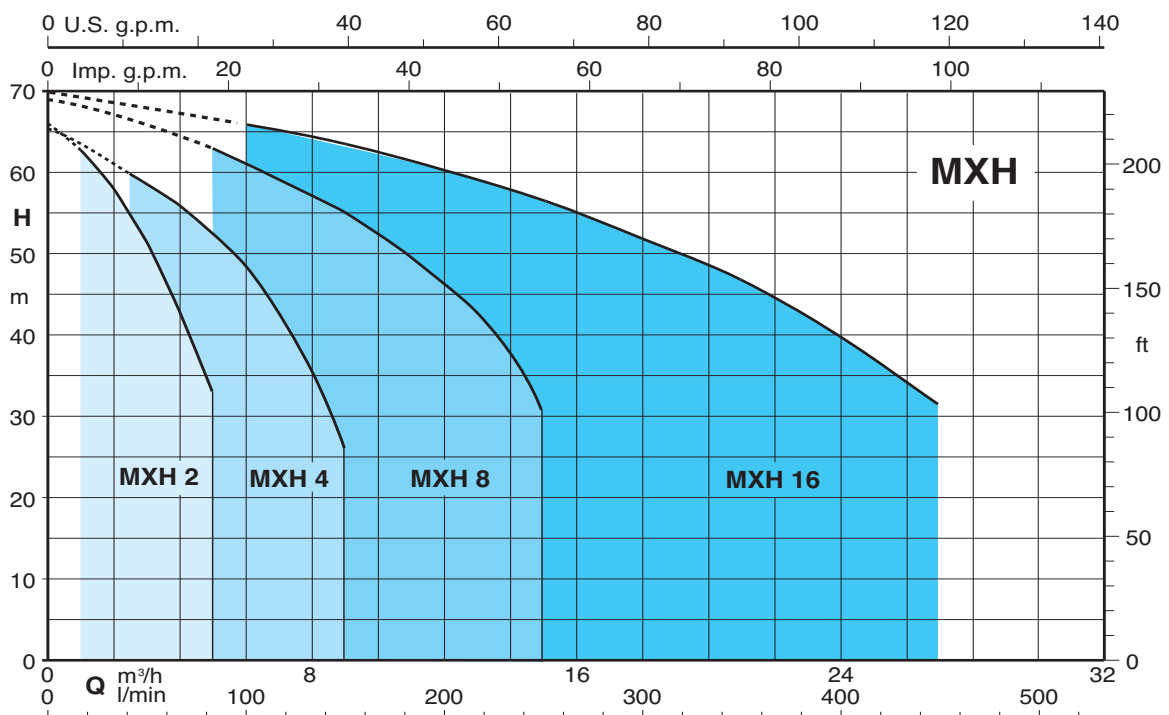
Coverage chart - Campo de aplicaciones n ≈ 3450 rpm
