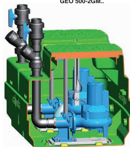
GEO 500-2GM..
