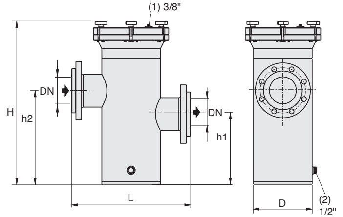
Flanges - Bidas
