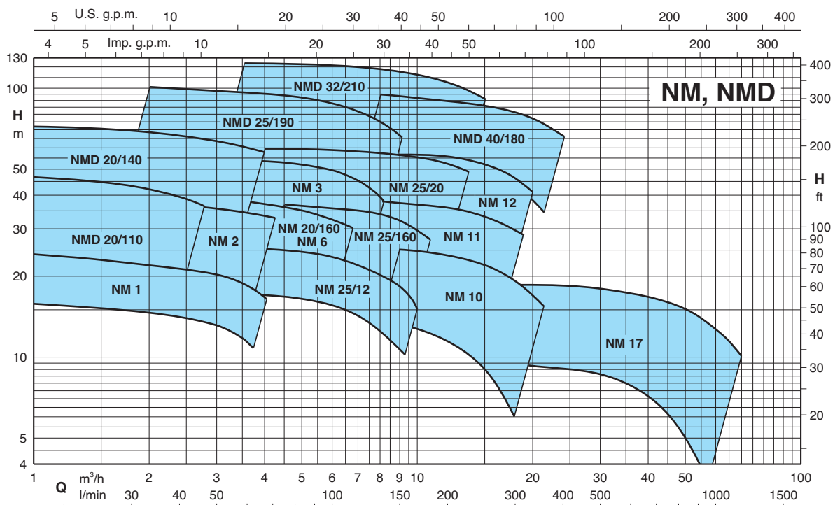
Coverage chart - Campo de aplicaciones n ≈ 3450 rpm
