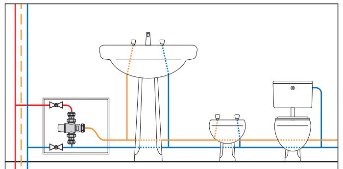
Прикладная схема смесителей серии 5213
