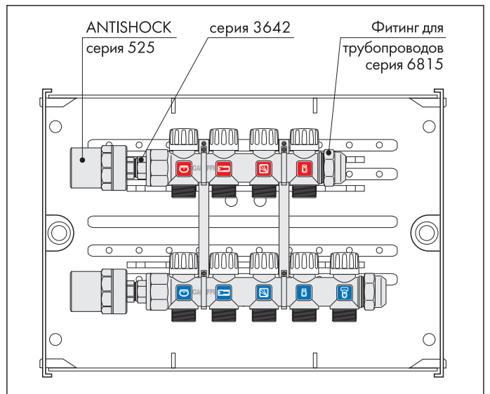
Пример состава распределительной установки
