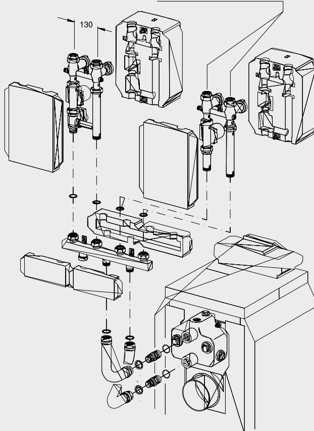
Подающая/обратная линии Rp1 для исполнения HS/HSM 25 и HSM 20; Rp1 1/4 для исполнения HS/HSM 32
