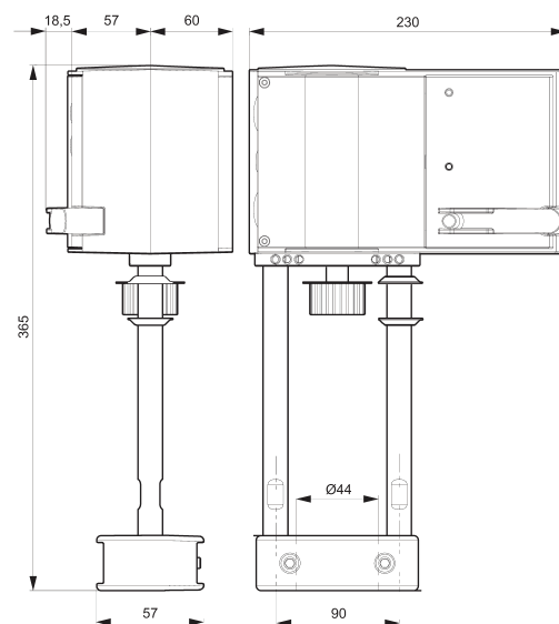
Габаритные размеры
