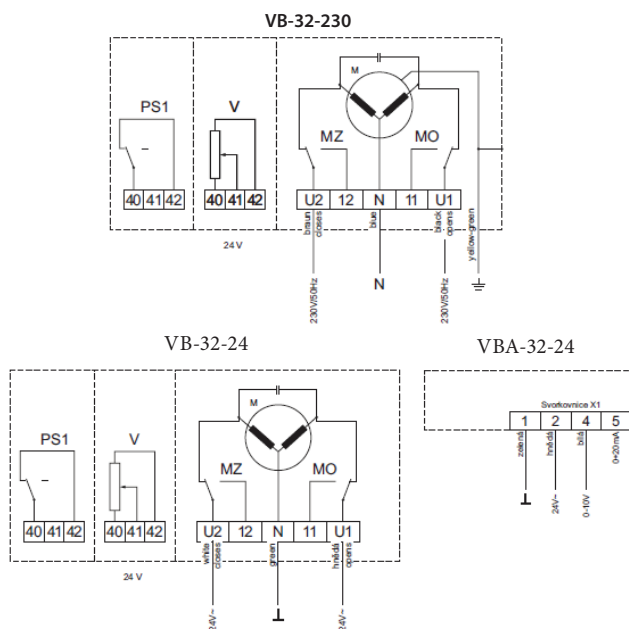
Подключение провода
