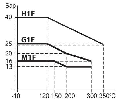
«Диagramma «Температура – Давление»
