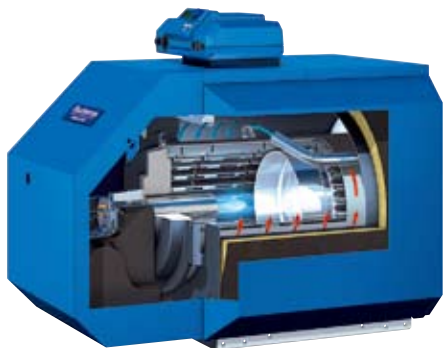
Работа горелки в котле
