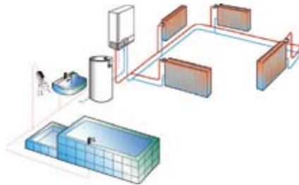
Система отопления с одноконтурным котлом и бойлером ГВС
