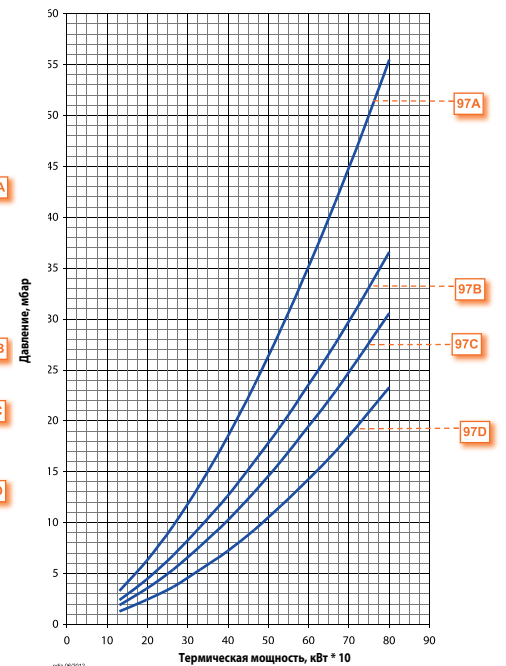
Потери напора (сопловая сборка + газовая рампа)
