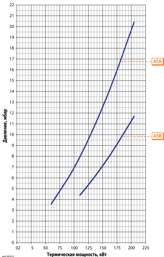
Потери напора (соловая сборка + газовая рампа)
