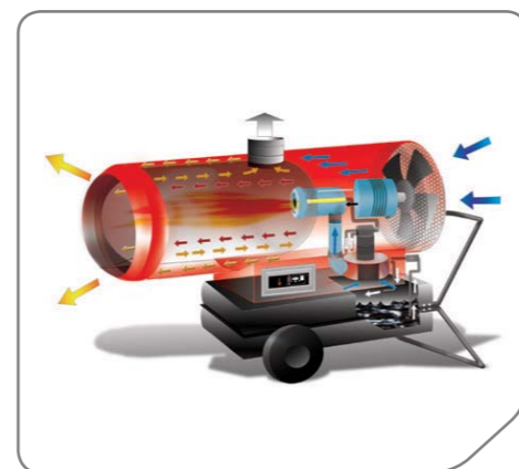
Принципиальная схема работы нагревателя серии PHOEN
