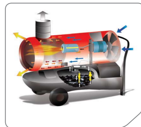
Принципиальная схема работы нагревателя серии ЕС
