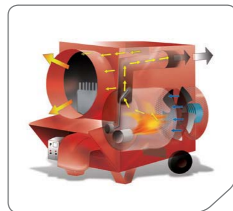
Принципиальная схема работы нагревателя серии JUMBO
