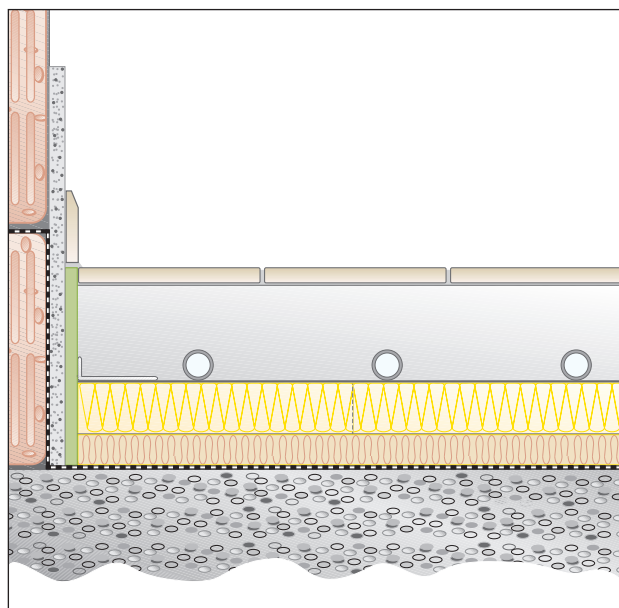
системный элемент валюфикс-рулон 35-3 перекрытия, граничащие с грунтом
